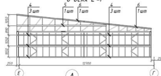
Схема наружной обрешетки в осях Е-Г
