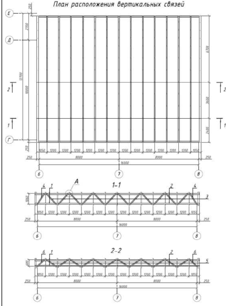
План расположения вертикальных связей
