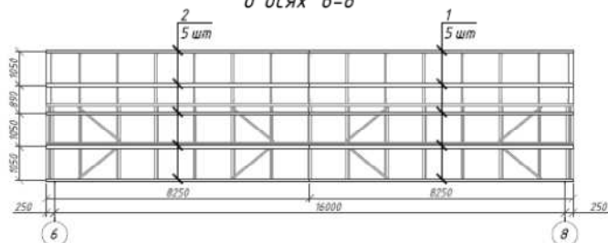
Схема наружной обрешетки в осях 8-6
