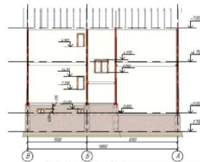
Срез Б-А
