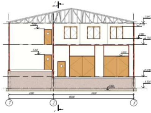
Срез Б-Б
