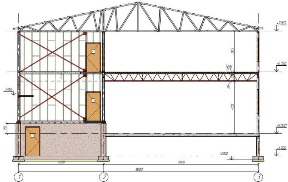
Разрез 2-2
