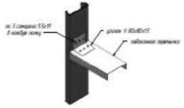
Узел крепления поперечной перемычки
